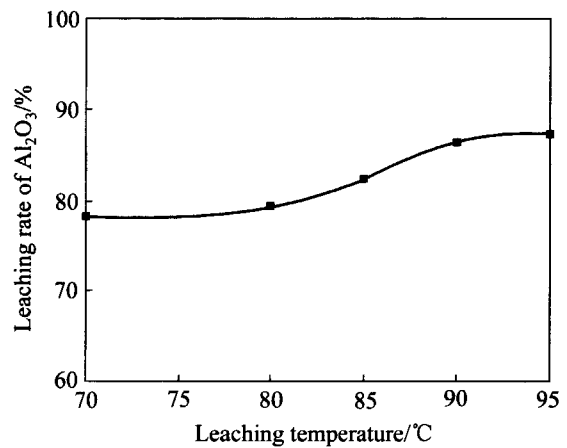
图 10 浸出时间为 2 h、碳酸钠用量为 120 g/L、氢氧化钠用量为 100 g/L 时浸出温度对 Al 2 O 3 浸出率的影响
