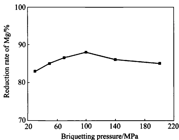
图7 还原剂过量系数为 5%、还原温度为 1 140 ℃、还原时间为 2 h 时制团压力对镁还原率的影响
