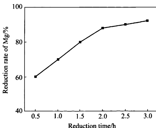
图5 铝粉过量系数为5%、制团压力为30MPa、还原温度为1140℃时还原时间对镁还原率的影响
