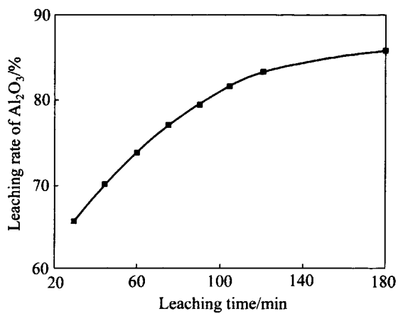
图 11 浸出温度为 95 °C、碳酸钠用量为 120 g/L、氢氧化钠用量为 100 g/L 时浸出时间对 Al 2 O 3 浸出率的影响
