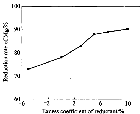
图6 制团压力为 30 MPa、还原温度为 1 140 ℃、还原时间为 2 h 时还原剂过量系数对镁还原率的影响
