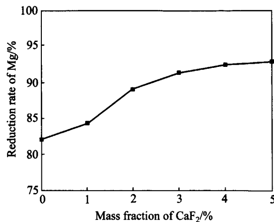
图8 还原剂的过量系数为 5%、制团压力为 30 MPa、还原温度为 1 140 ℃、还原时间为 2 h 时 CaF 2 添加剂对镁还原率的影响
