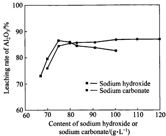
图 12 浸出温度为 95 °C、浸出时间为 2 h 时氢氧化钠和碳酸钠浓度对 Al 2 O 3 浸出率的影响
