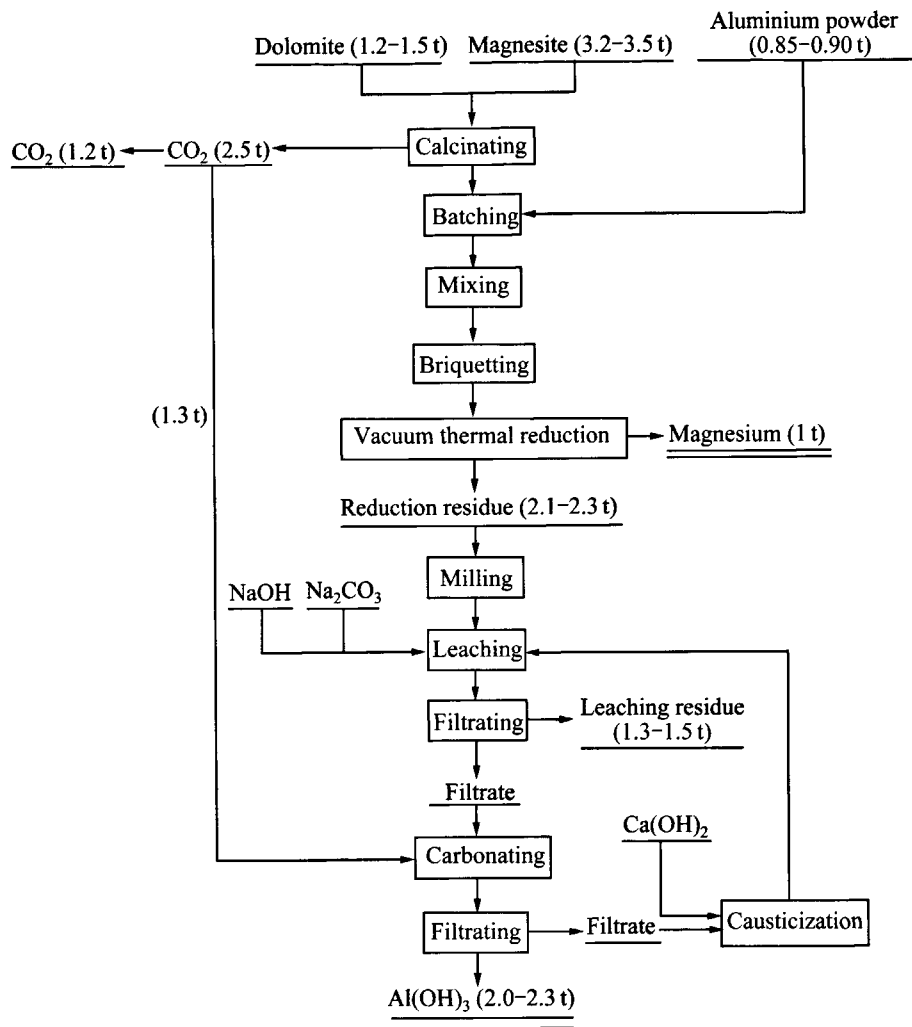
图2 新法炼镁工艺流程和物料平衡
